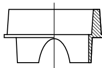
Fig. No. 6016-SQ 2 1/4" Square Adapter
